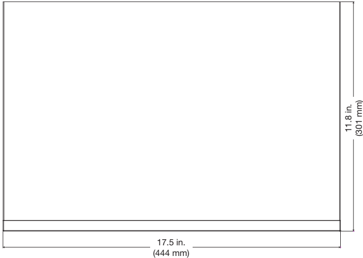
GE-DS-242-PoE
